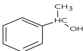
1-fenil etanol
