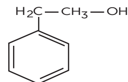
2- fenil etanol
