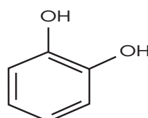
1,2 dihidroxifenol
